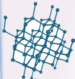
Алмаз
