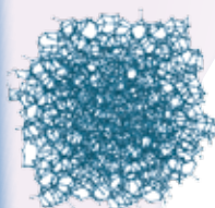
Сажа
