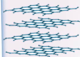
Графіт
