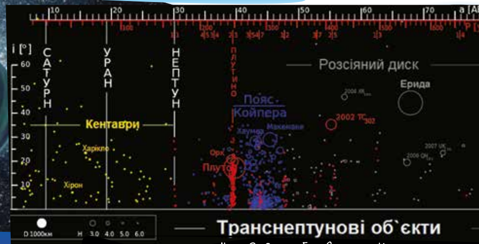
Мал. 3. Схема будови поясу Койпера.
