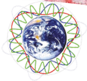
Мал. 1. Зростання середньої температури на поверхні Землі
