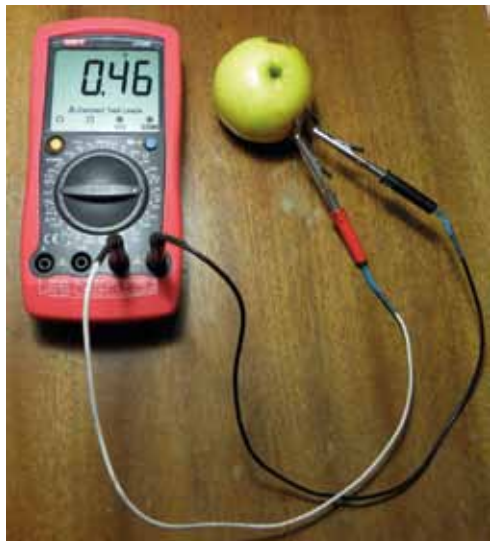
Мал. 3. „Яблучний” гальванічний елемент
