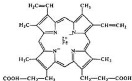
Мал. 5. Структурна формула хлорофілу а (А) та гему гемоглобіну (Б)
